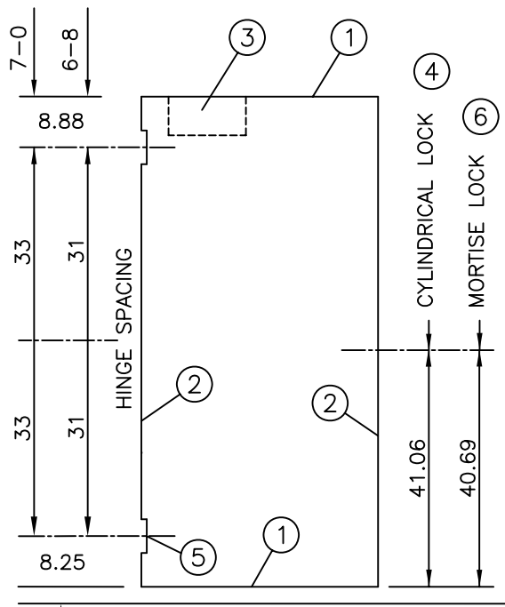
DOOR ELEVATION
