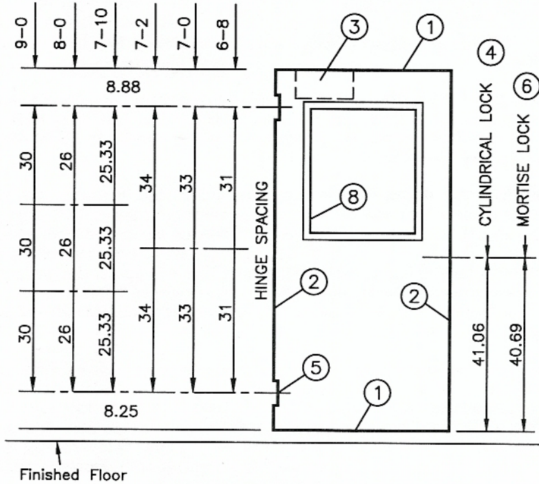
DOOR ELEVATION
